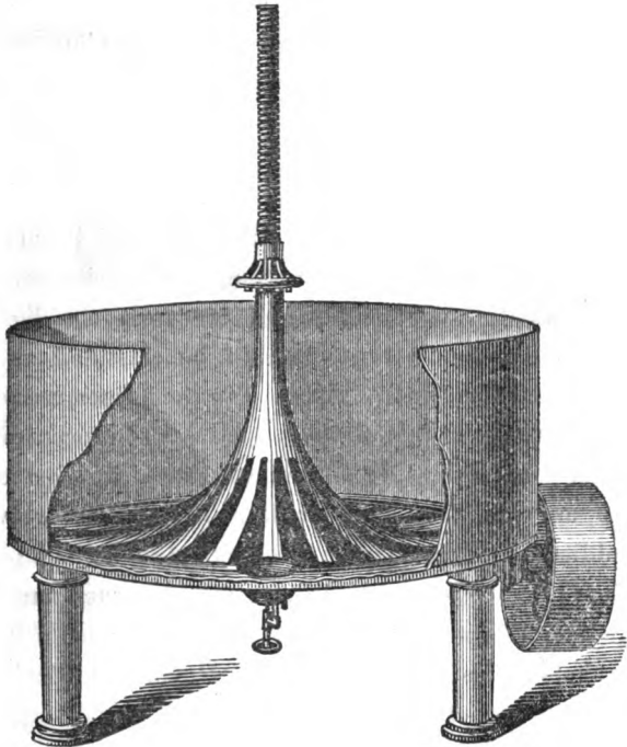
CONOIDAL SEPARATOR.
